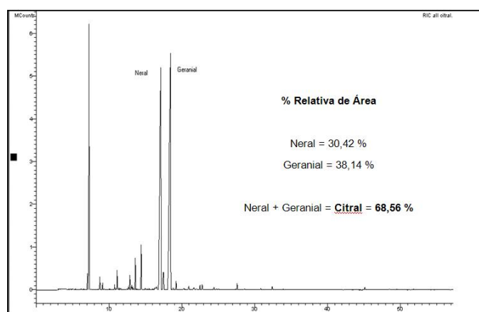
Figura 1. Cromatograma do óleo essencial do Cymbopogon citratus . Os Tempos de retenção para o Neral e Geranial foram 17,07 e 18,40 minutos, respectivamente.
