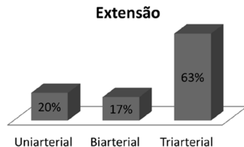
Gráfico 2. Distribuição da AC e sua extensão.
