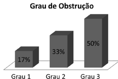
Gráfico 1. Distribuição dos graus de obstrução.
